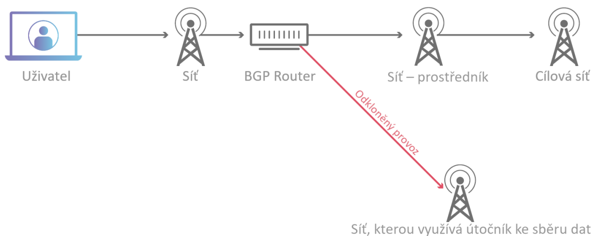
Obrázek 2: Schéma útoku na protokol BGP s cílem odklonění komunikace
